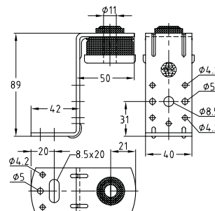
Luchtkanaal-dubbelhoek Type II
