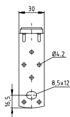
Luchtkanaal-hoek Type I
