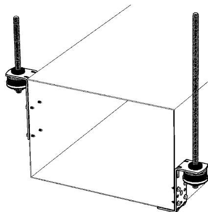
Luchtkanaal-hoek
