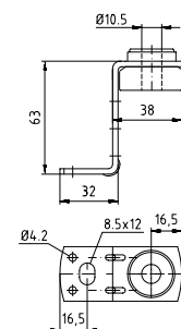
Luchtkanaal-dubbelhoek Type I
