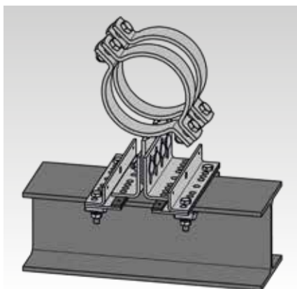
Type FG, met glijplaat
