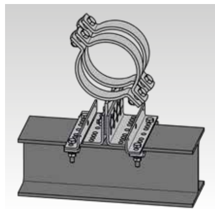
Type F, zonder glijplaat
