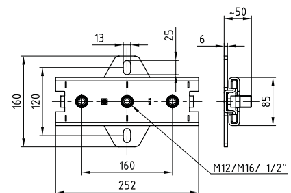
Montage von zwei Schraubrohrschele mit Anschlussgewinde M16 auf einer MPT-Konsole, Q100
