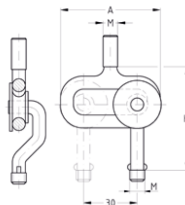
Bevestiging aan een MPC Systeemrail
