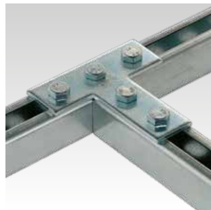
T-Verbindingsplaat
