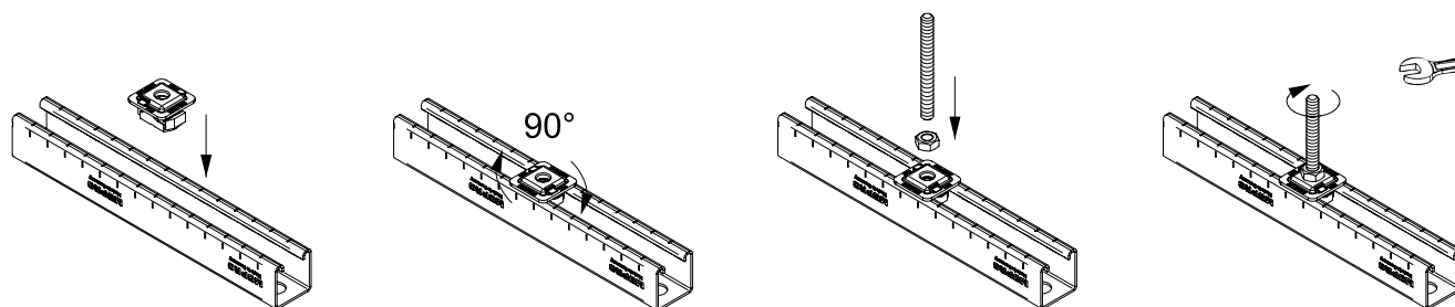
Uitvoering M16 + R \frac{1}{2} "
