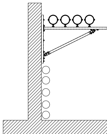
Montage de tuyauteries sur une console et une jambe de force
