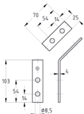
Montagehoeken 45°
