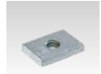
Größe 38/24-40/120
