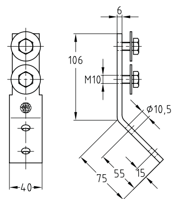
Equerre 45°
