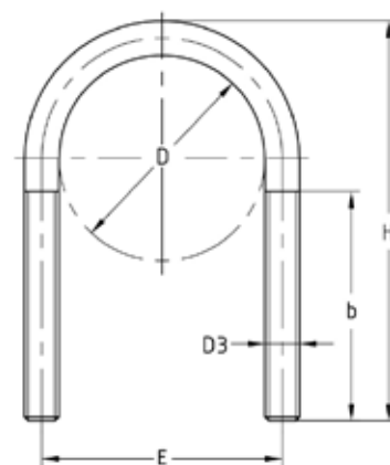
Ausführung M8 bis M12 mit Muttern und Unterlegscheiben
