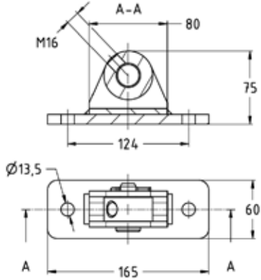
Ausführung M16
