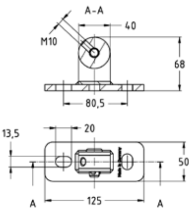
Ausführung M10
